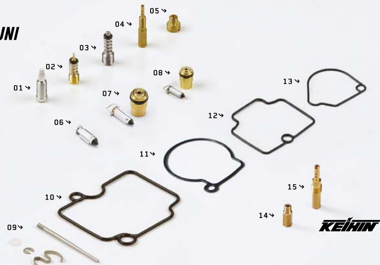
VÝPUSTNÍ ŠROUBEK KARBURÁTORU MIKUNI® MIKUNI® TANK SCREW
