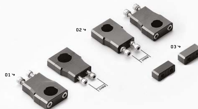
DRŽÁKY ŘÍDÍTEK YCF 2012-2019 BAR MOUNTS FOR YCF 2012-2019
