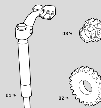
OVLÁDACÍ HŘÍDELKA SPOJKY PUSH ROD
